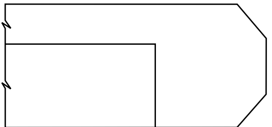
DOUBLE BEVEL
